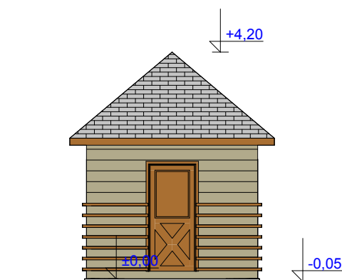
ELEWACJA POŁUDNIOWO - ZACHODNIA
