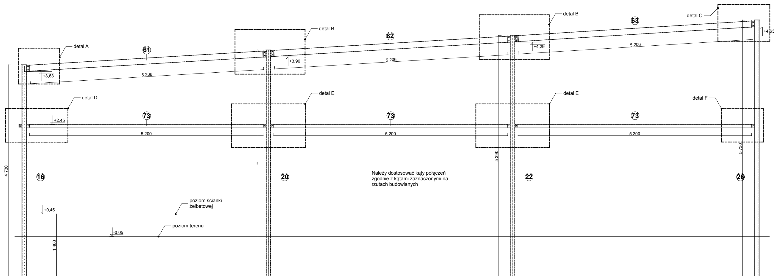
SCHEMAT UKŁADU SŁUPÓW I BELEK, SKALA 1:50
