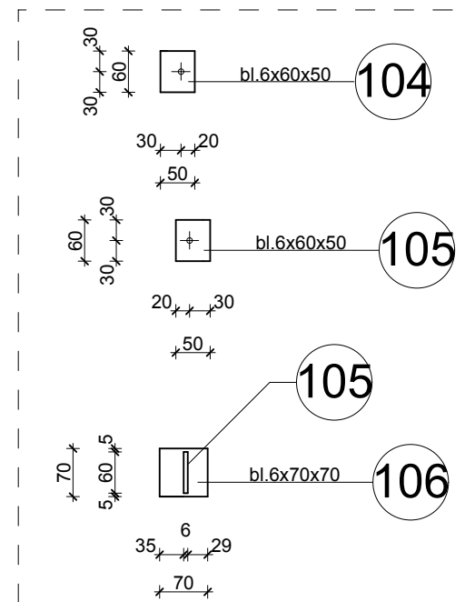
DETAL POŁĄCZEŃ, SKALA 1:10
