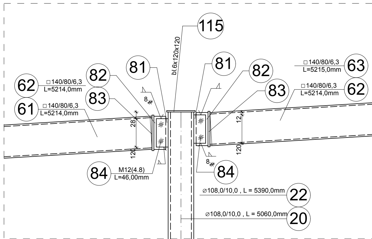
DETAL B, SKALA 1:10
