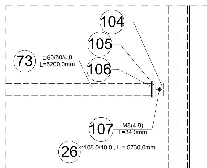
DETAL F, SKALA 1:10
