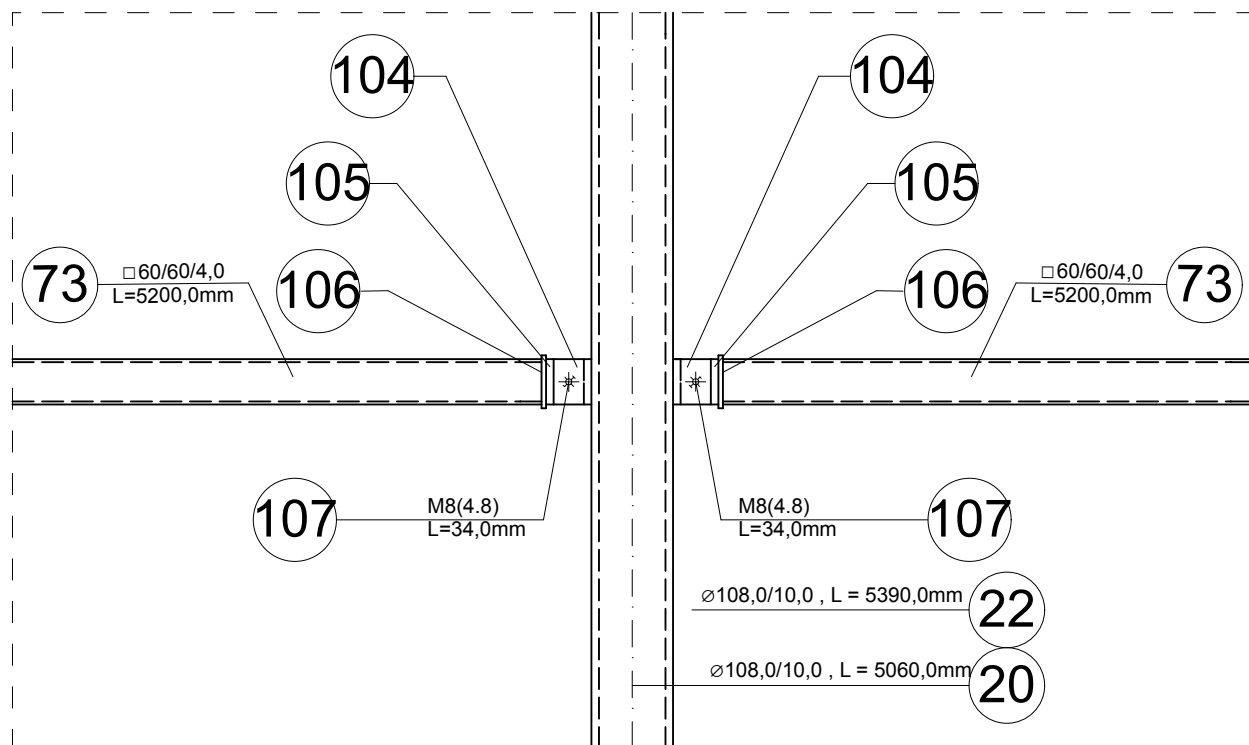
DETAL E, SKALA 1:10
