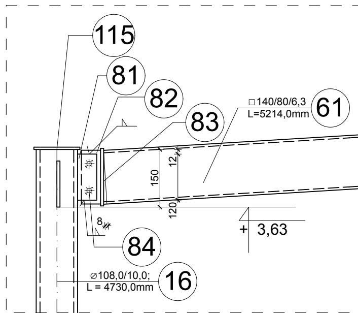
DETAL A, SKALA 1:10
