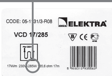
Заводская наклейка
