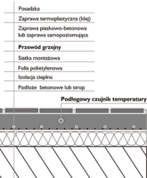
Rys. 3c Przekrój podłogi przy zastosowaniu siatki montażowej
