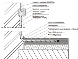
Rys. 3b Montaż regulatora temperatury z czujnikiem podłogowym
