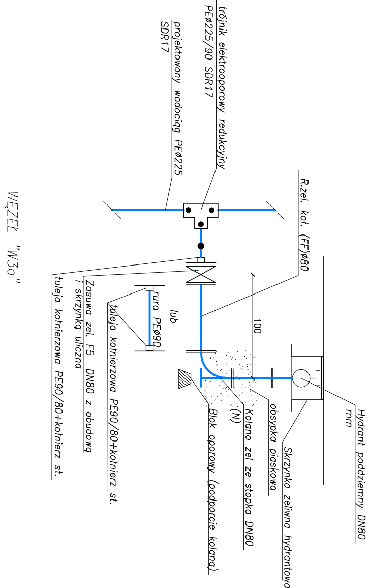
SCHEMAT WPIĘCIA HYDRANTÓW DO WODOCIAGU PEØ225
